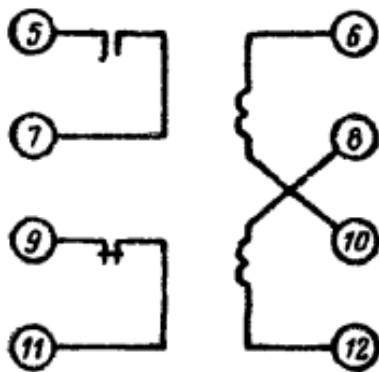
Рис. 2-40. Схема внутренних соединений реле РТ-40.
