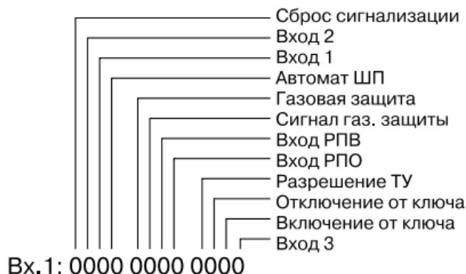
Расписание входных дискретных сигналов устройства в режиме «Контроль»
